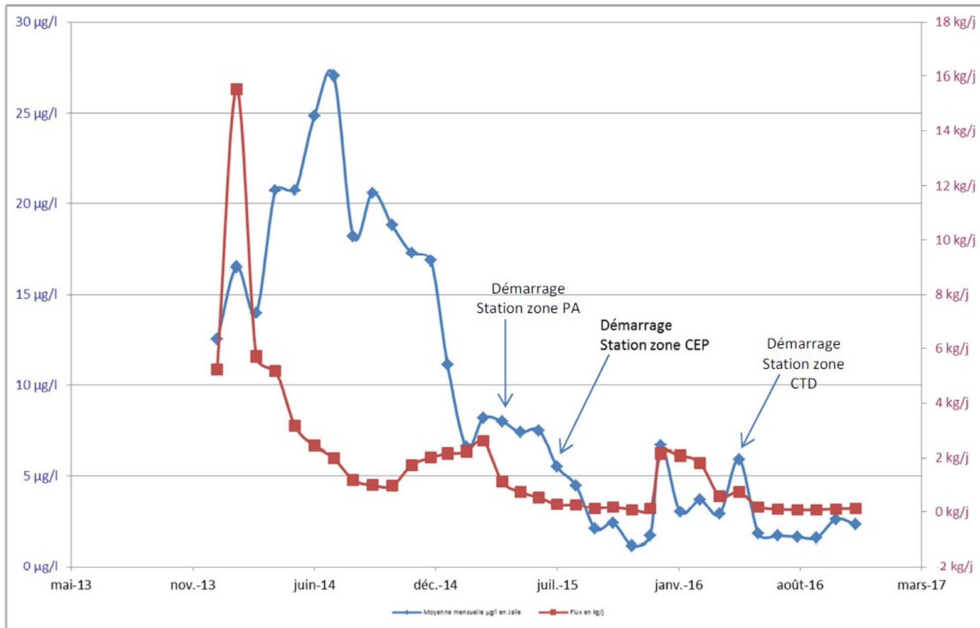
Evolution de la concentration en perchlorate dans le cours d'eau Jalles de Blanquefort à l'aval de la plate-forme (et évolution du flux de perchlorate présent dans ce cours d'eau ayant pour origine la pollution des nappes souterraines)
